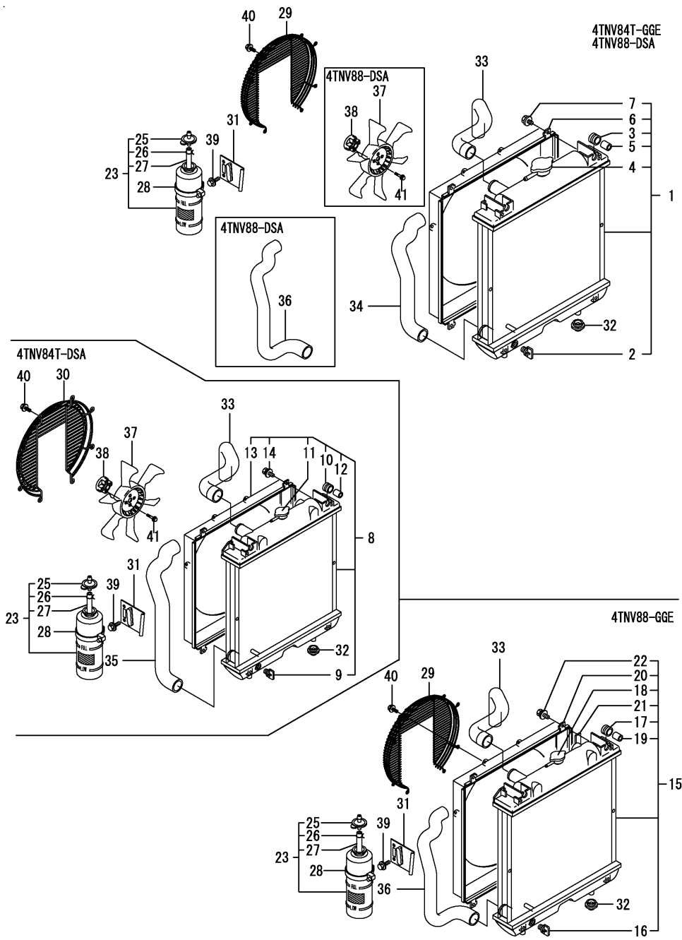
Fig.7. RADIATOR
