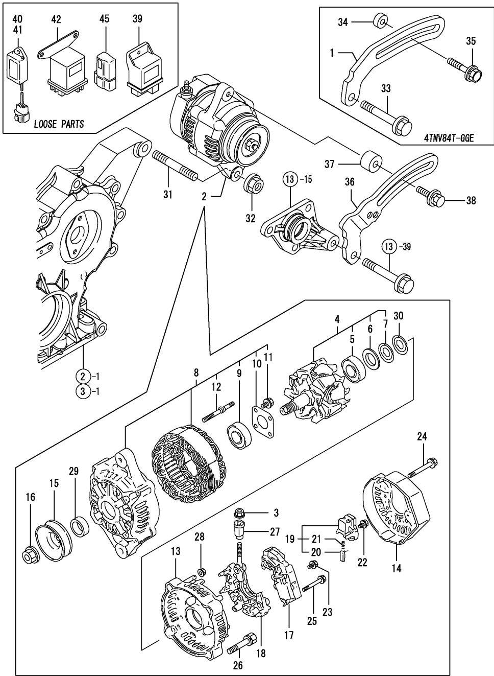
Fig.21. GENERATOR
